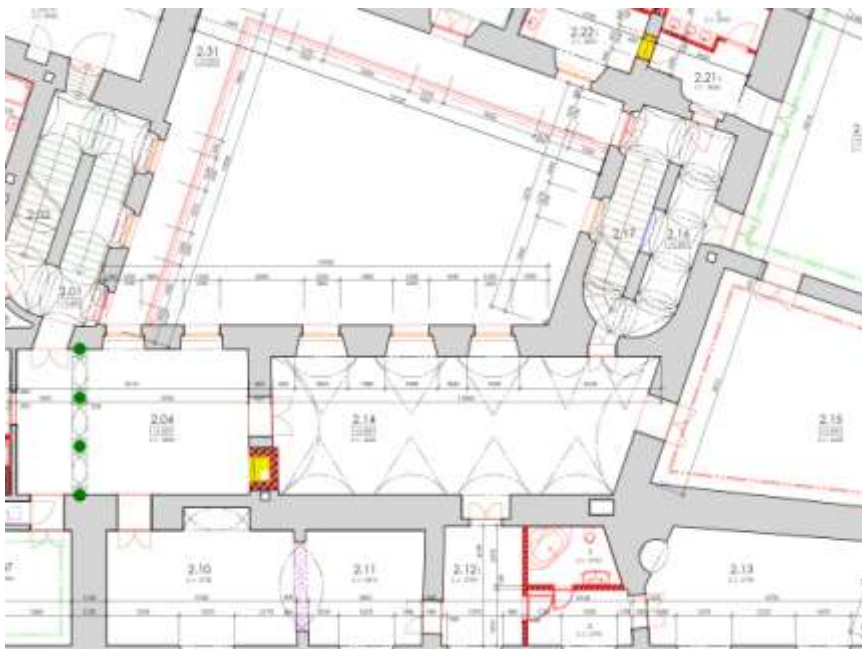
3. Bono Publico – ukázka projektu 2. nadzemního podlaží zámku
