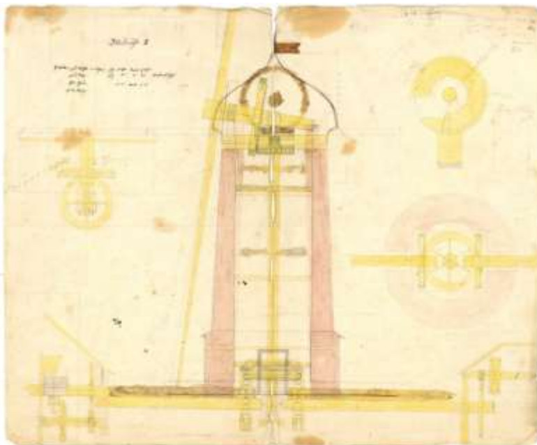
Nákres větrného mlýnu na Věteráku
