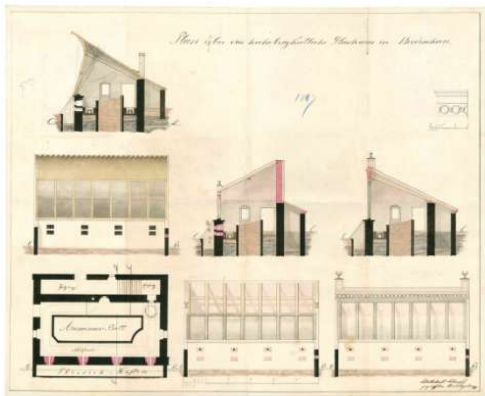
Nákres zámeckého skleníku
