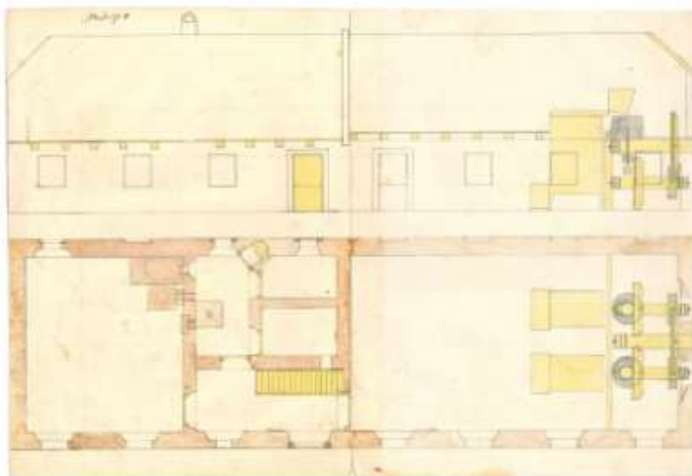
Nákres hospodářské budovy propojené s větrným mlýnem
